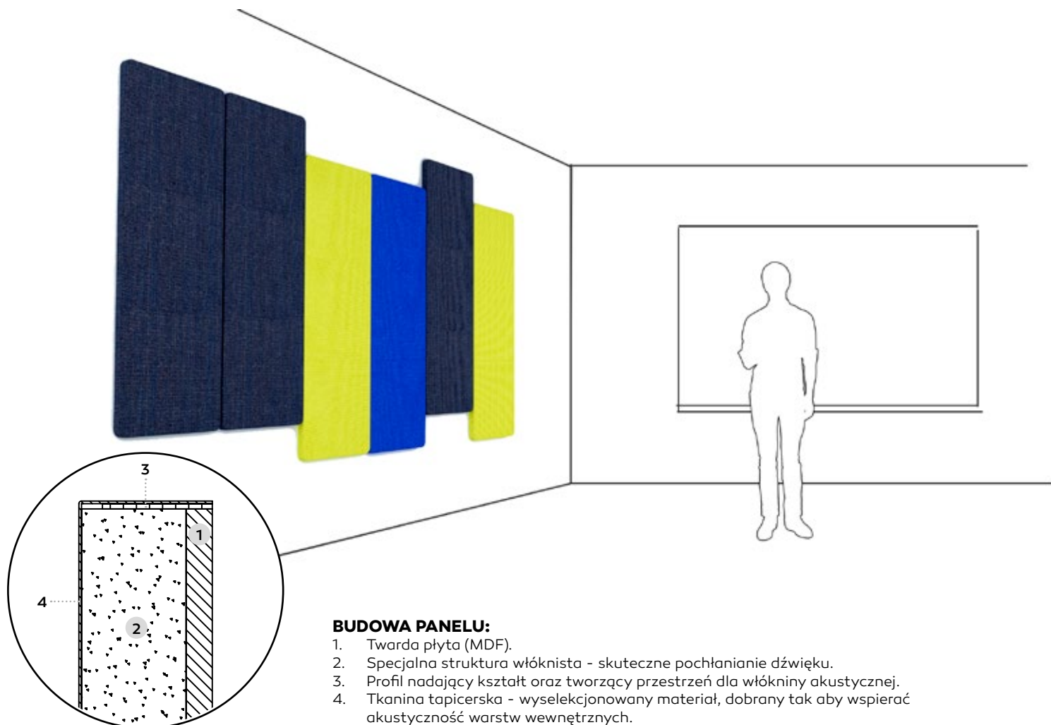
Przekrój panelu akustycznego SELVA WALL
